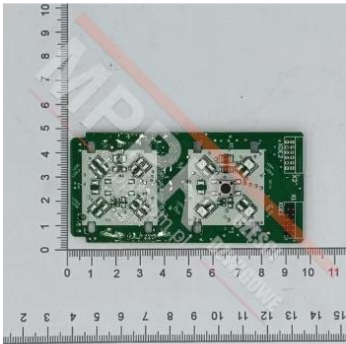
59324332 PCB for LCS PCBA LOPDA1.QB
