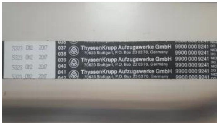
99000009241 Pas zębaty L=1570mm zamknięty Thyssen
