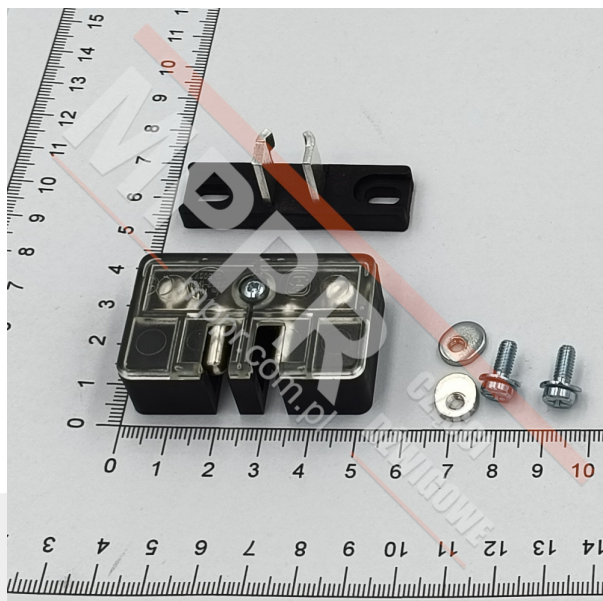
Kontakt elektryczny AZ02 ze zworką dla rygla BKG
