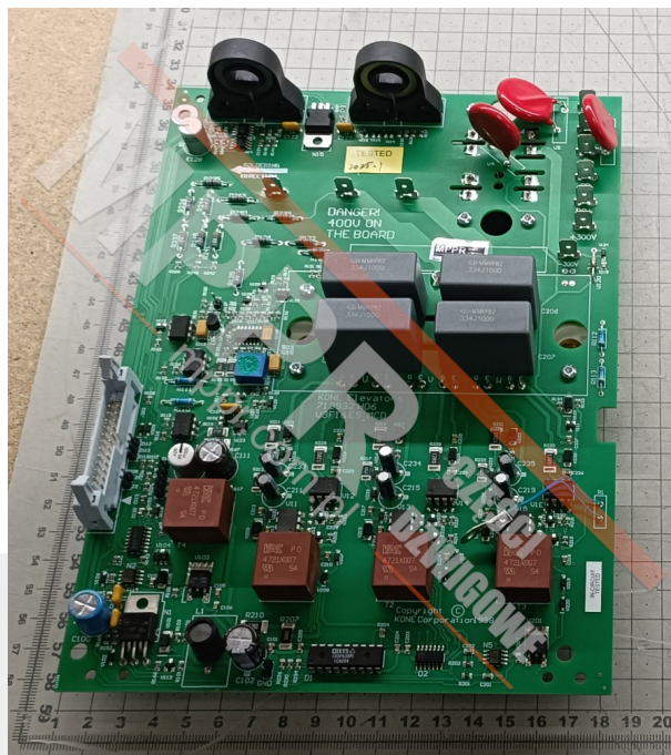
KM713930G01 Płyta główna LCE dla falownika V3F16
