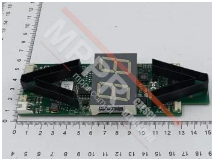
594234 Płytki SLINV 51.Q wyświetlacza położenia kabiny do dźwigu Schindler
