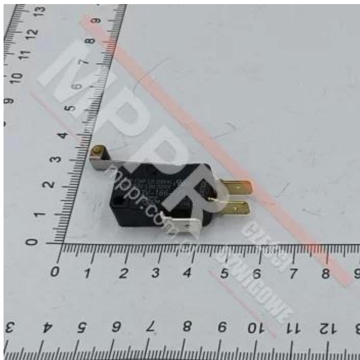
927072 Mikroprzełącznik do QKS11; 16 A, 250 V, 1CO
