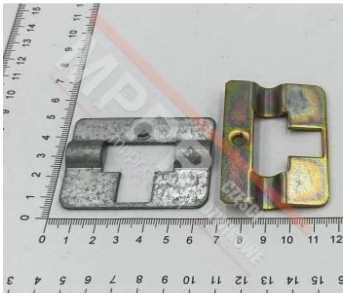
AGH.0006.C00000 Suwaki drzwi szybowych, 2 szt.
