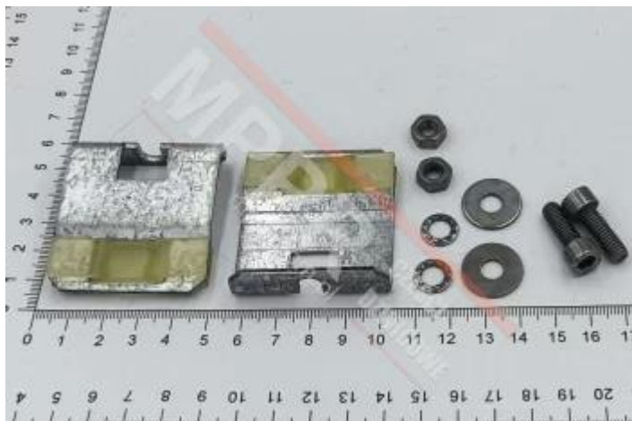
AGH.03B0.00000 Kompletne suwaki 8 mm drzwi, 2 szt.
