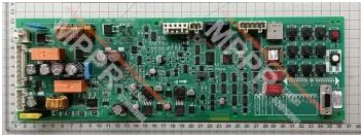
Płyta SPBC (Service Panel Board CAN) OTIS
