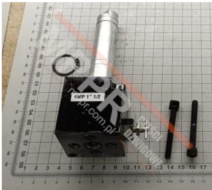
Zawór elektromagnetyczny VMP 1½"
