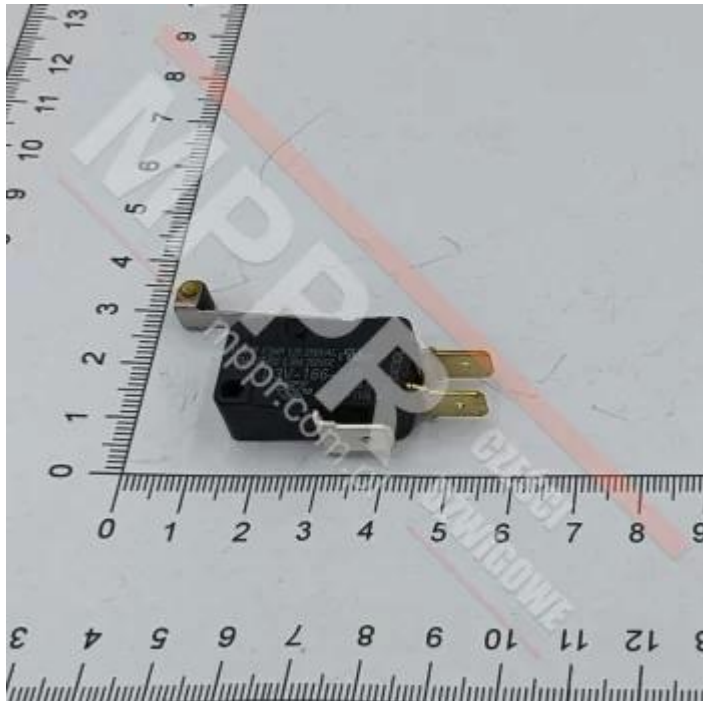
Mikroprzełącznik do QKS11; 16 A, 250 V, 1CO
